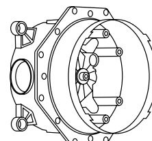
iBox® universal Runko-osa iBox universal # 01800180 Jatkoholkki 25 mm liian syvällä asennuksella: # 13595000 Jatkoholkki 22 mm liian pienellä asennussyvyydellä: # 13597000 Ecostat S:lle, halkaisija 150 mm # 15497000 Ecostatille 155 x 155 mm # 15597000 Ecostat E:lle ja PuraVidalle 155x155 mm # 13596000 peitelaipoille halkaisijaltaan 170 mm
