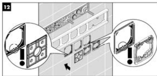
Pintaosien esiasennus
