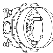
iBox® universal Runko-osa iBox universal # 01800180 Jatkoholkki 25 mm liian syvällä asennuksella: # 13595000 Jatkoholkki 22 mm liian pienellä asennussyvyydellä: # 13593000 ShowerSelectille halkaisijaltaan 155 mm x 155 mm # 13597000 ShowerSelectille halkaisijaltaan 150 mm # 13601000 ShowerSelectille integroidulla pidikkeellä # 13604000 ShowerSelectille lasipinnalla
