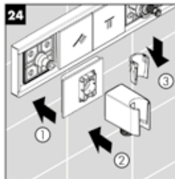
Asenna letkuliitin-pidike paikoilleen
