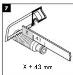
Letskuliittimen nipan lyhen- täminen. Mittaa tarkasti
