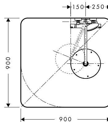
Asennus: suihku
