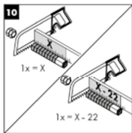
Käyttöventtiiliin ja termo- staattielementin kiinnikkei- den lyhentäminen
