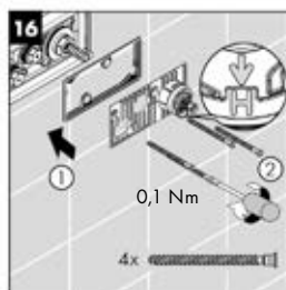
Kiristä termostaattiele- mentin ruuvit, vääntömo- mentti 0,1 Nm
