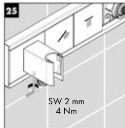
Kiinnitä letkuliitin-pidike, vääntömomentti 4 Nm
