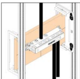
Asennus kannatinjärjestelmään
