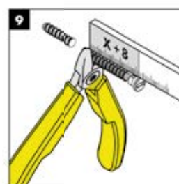
Kiinnitysruuvien katkaisu. Mittaa tarkasti
