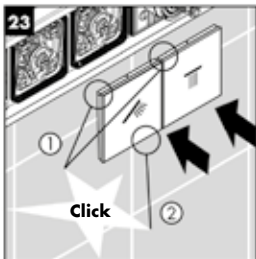
Napsauta oikeat painikkeet paikoilleen
