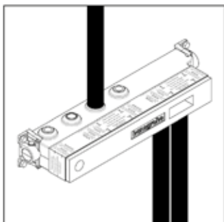
Asennus suoraan seinään
