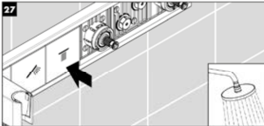
Testaa yläsuihkun painikkeen toiminta
