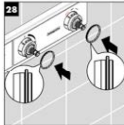
Asenna pintapeitelevy ja tiivisterenkaat
