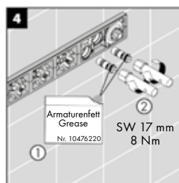
Asenna äänieristeet, takaiskuventtiilit ja roskasihdit
