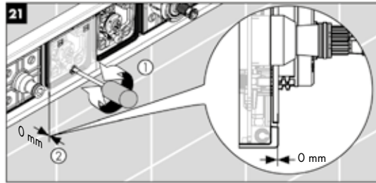
Säädä asennusapukappale sopivalle korkeudelle
