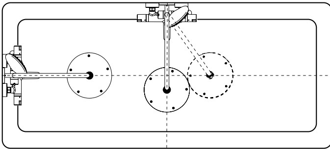
Asennus: amme
