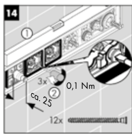
Kiristä Select-säätöosien ruuvit, vääntömomentti 0,1 Nm
