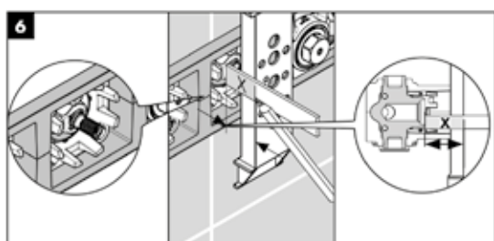
Mittaa liittimille, kiinnikkeille ja ruuveille optimaalinen pituus aputyökalun avulla. Mittaa tarkasti
