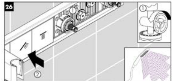
Avaa vedentulo ja testaa käsisuihkun painikkeen toiminta
