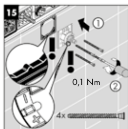
Kiristä käyttöventtiilin ruuvit, vääntömomentti 0,1 Nm
