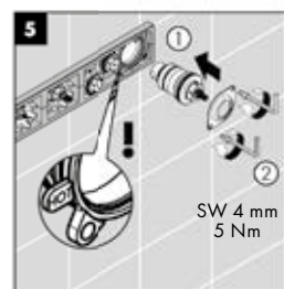
Asenna termostaattiele- mentti
